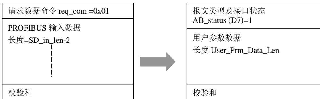
图 4-9 用户模板发一输入数据报文 req_com=0x01，接口板答一输出数据报文格式 B
