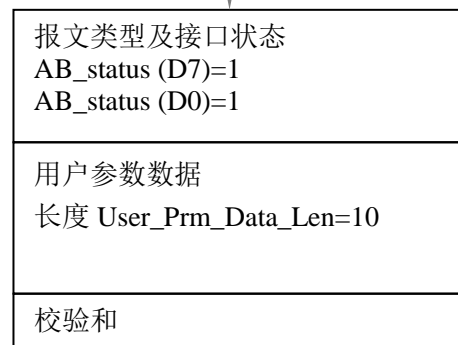
图 4-21-5 接口板回答报文格式 B，AB_status (D7)=1 且 AB_status (D7)保持 1。
