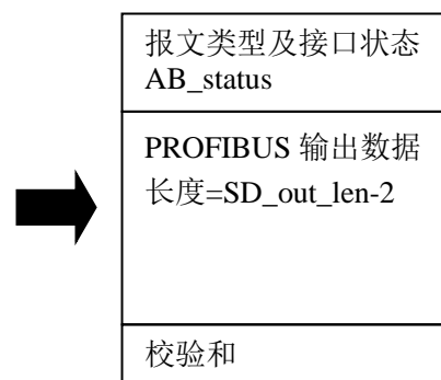
图 4-12 接口板回答输出数据报文格式 A
