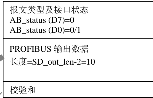
图 6-6-2 接口板回答输出数据报文格式 A，且 AB_status (D7)=0
