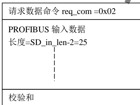
图 4-21-6 用户板发 req_com=0x02，清除 AB_status (D0)=1，准备接收格式 A
