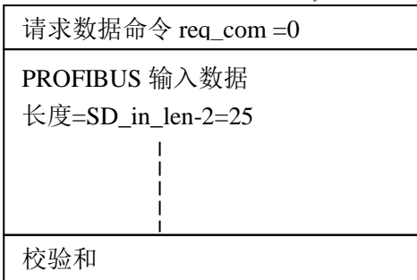
图 6-6-3 用户板判断 AB_status (D0)=0 继续发 req_com =0，接收格式 A
