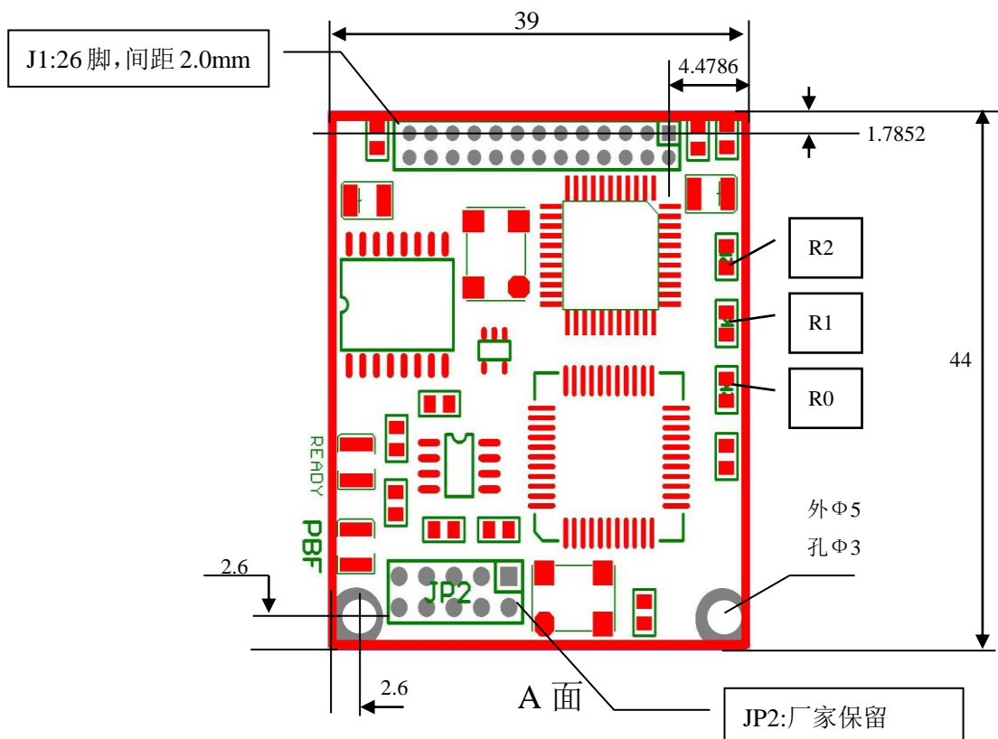
图 3-3 PB-OEM2-SEH 产品尺寸图
