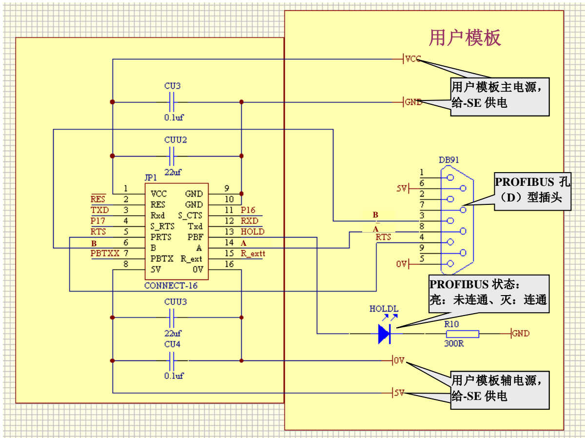
图 3-12 连接方式 0—PB 的 D 型插座 PROFIBUS 信号来自 J1-16
