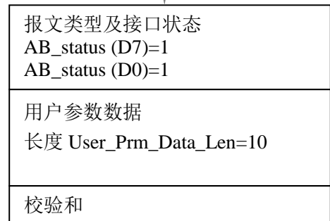
图 6-6-5 接口板回答报文格式 B，AB_status (D7)=1 且 AB_status (D7)保持 1。
