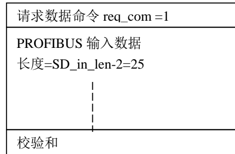
图 6-6-4 用户板判断 AB_status (D0)=1 发 req_com =1，接收格式 B
