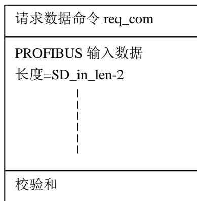
图 4-7-1 用户模板发一输入数据报文格式
