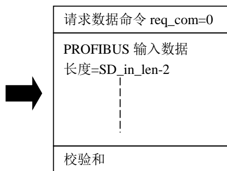
图 4-11 用户板发输入数据报文中 req_com=0
