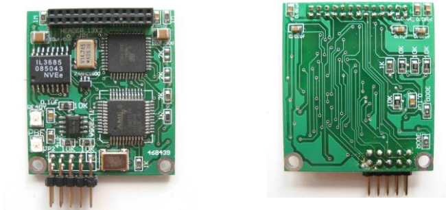
图 3-2 PB-OEM2-SEHH 产品外形
