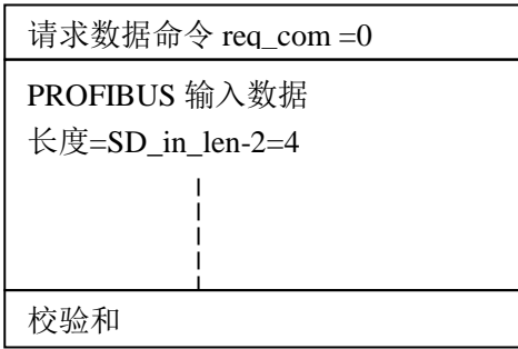
图 6-6-1 使用用户参数功能条件下，用户板首先发请求数据命令 req_com 0
