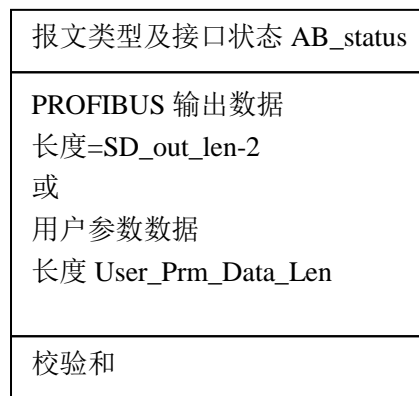
图 4-7-2 接口板答一输出数据报文格式
