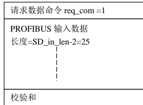
图 4-21-4 用户板判断 AB_status (D0)=1 发 req_com =1，接收格式 B
